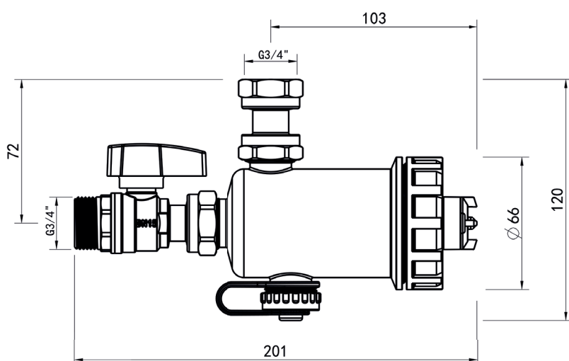
Defangatore
