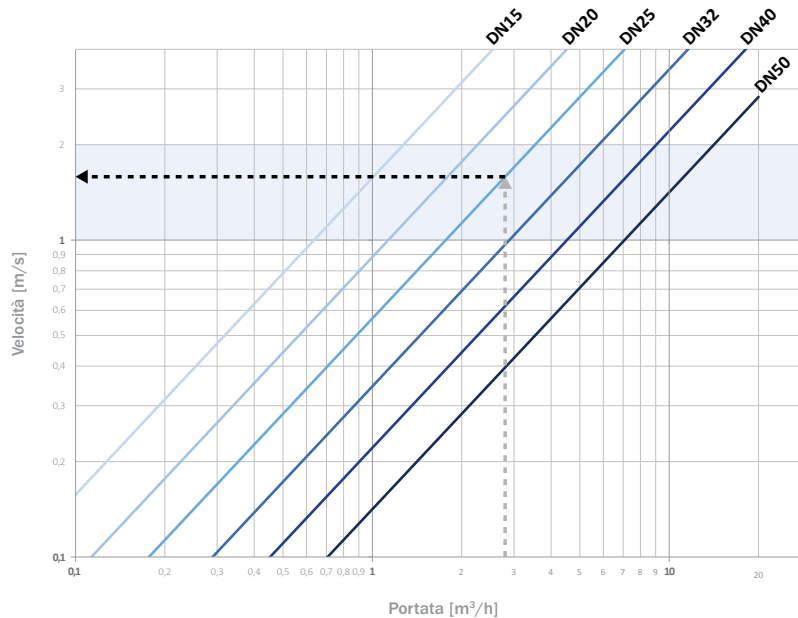
DIAGRAMMA PORTATA - VELOCITÀ
