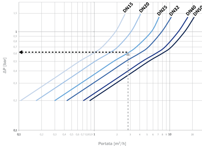
DIAGRAMMA PORTATA - ΔP
