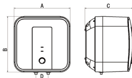
Figura 3 – Modello 10-15 LT sopra lavello
