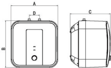
Figura 4 – Modello 10-15 LT sotto lavello
